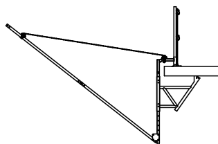
914014 Safety Fan Slab
